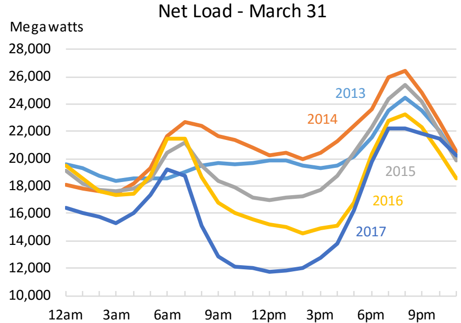
CAISO - Actual
